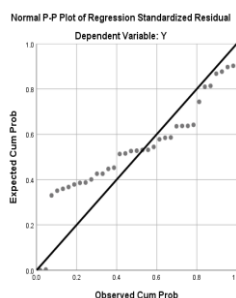
Gambar 5. Grafik Normalitas
